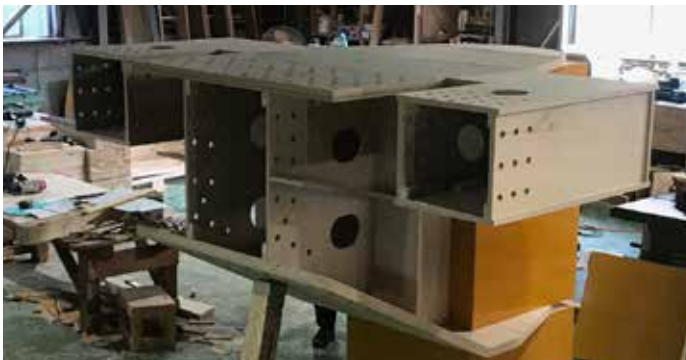
鋼桁モックアップ
